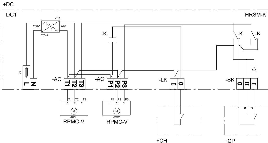
Fig. 39 Wiring diagram HRSM-K
